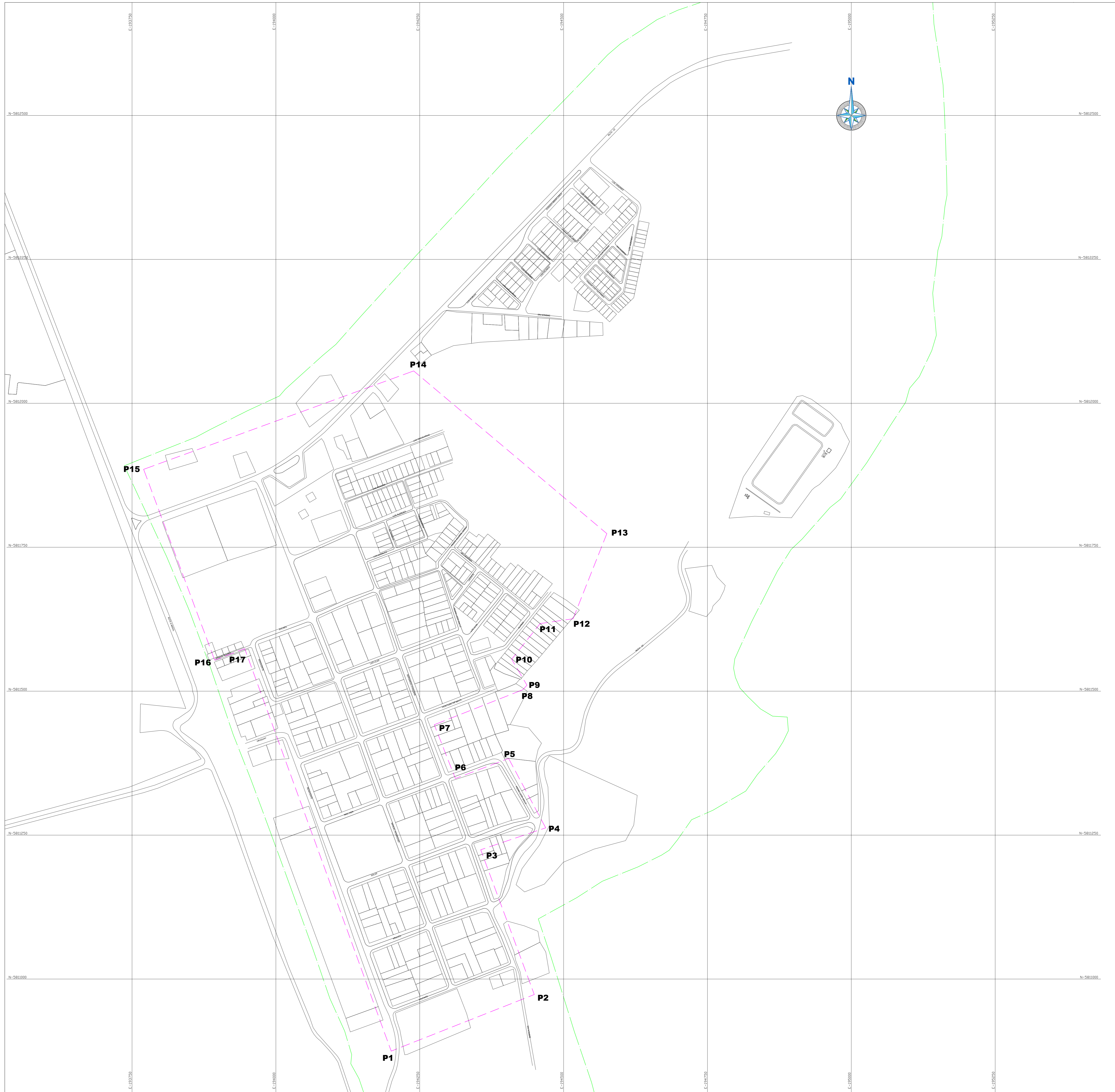
PLANTA GENERAL DE MININCO TERRITORIO OPERACIONAL ESCALA 1:2500
